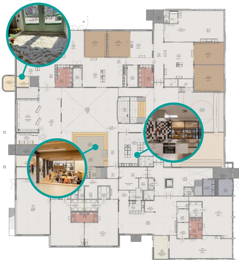
Begane grond
